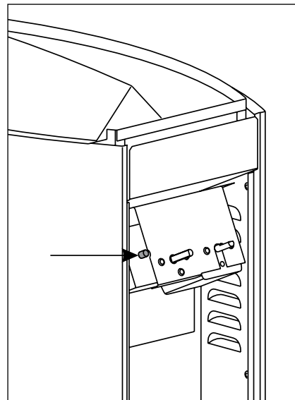
Kuva 12. Ylikuumenemissuojan palautuspainike Bild 12. Överhettningsskydd
