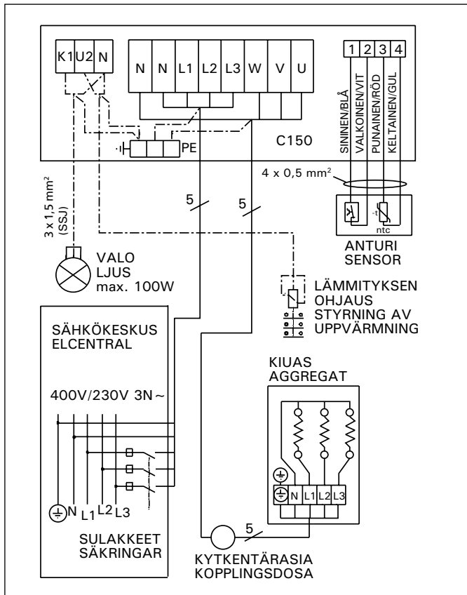
Kuva 11. Ohjauskeskuksen C150 ja BCE-kiukaan sähkökytkennät Bild 11. Elinstallationer av styrenhet C150 och BCE-aggregat
